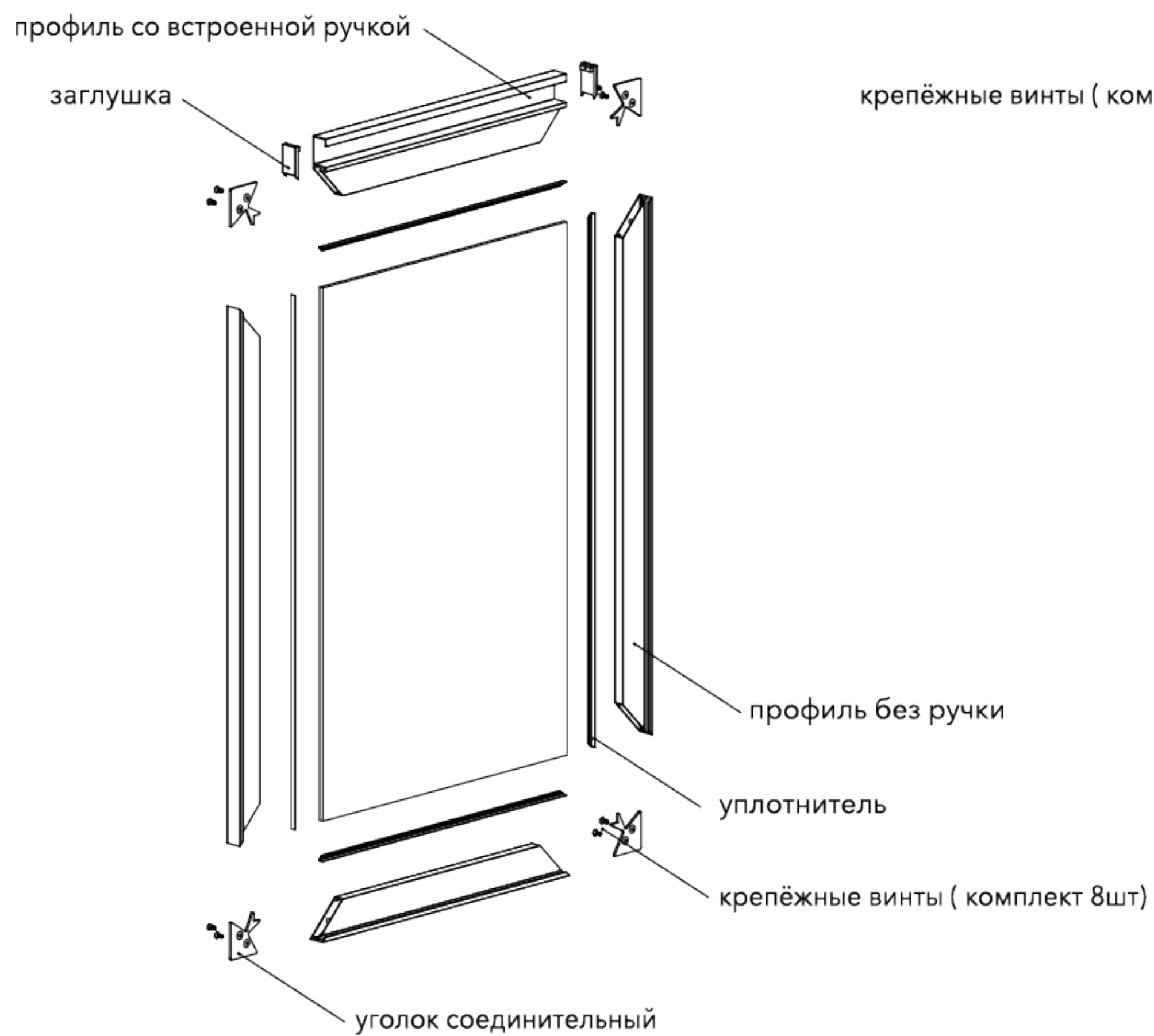
Схема сборки фасада с горизонтальной планкой со встроенной ручкой
