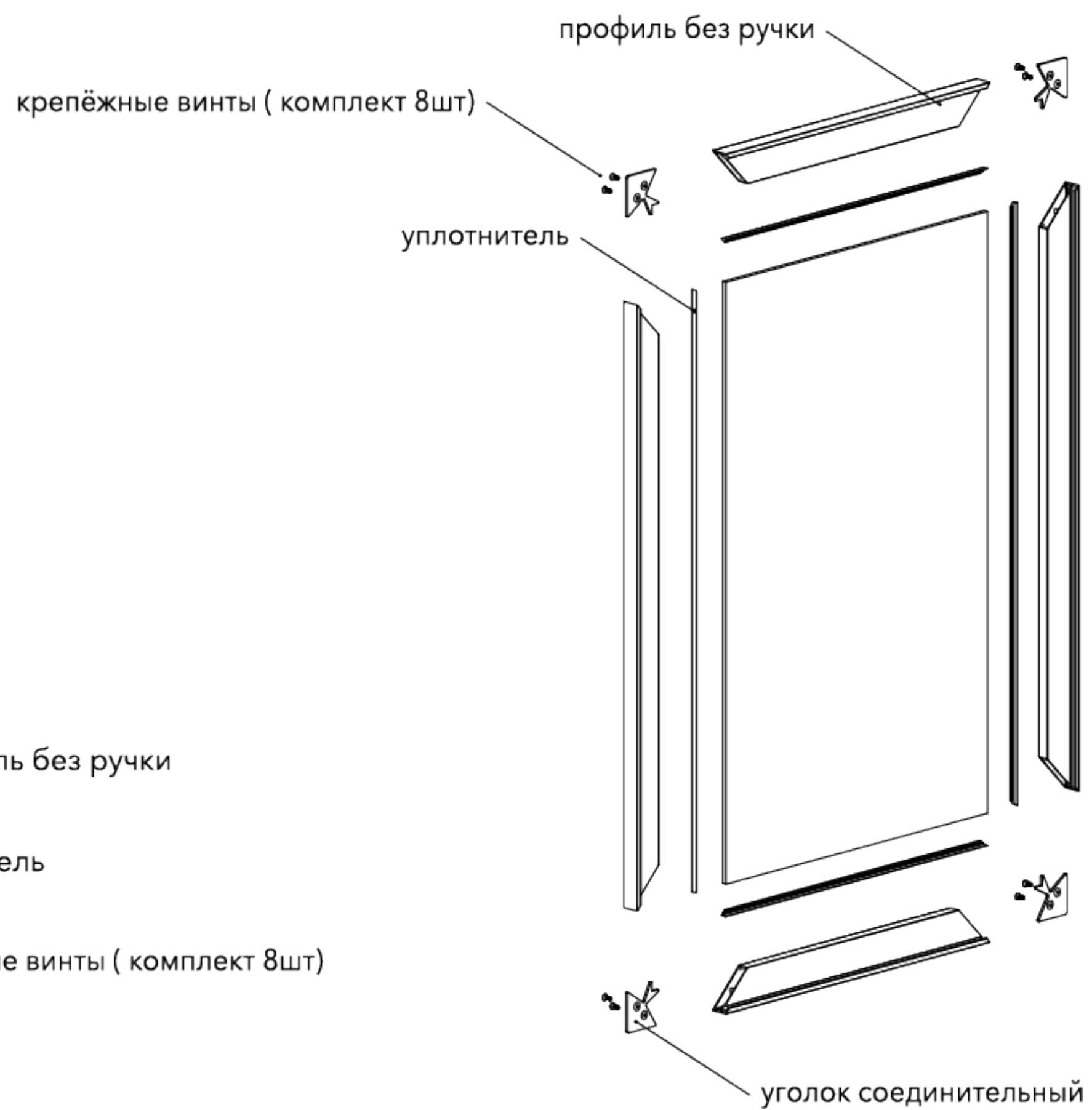
Схема сборки фасада без встроенной ручкой
